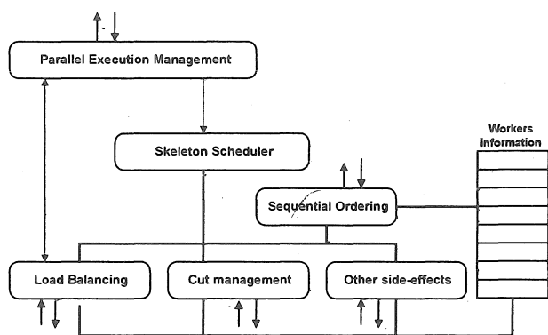
FIGURA 1 Organização interna do escalonador
