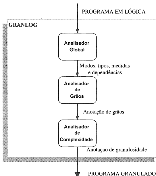
FIGURA 3 - Visão dos módulos do GRANLOG
