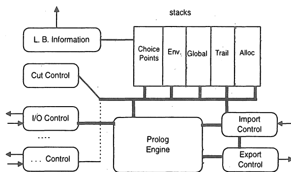
FIGURA 2 Organização interna do trabalhador
